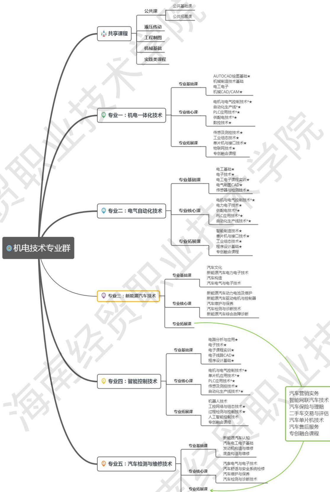
图2 课程结构图
